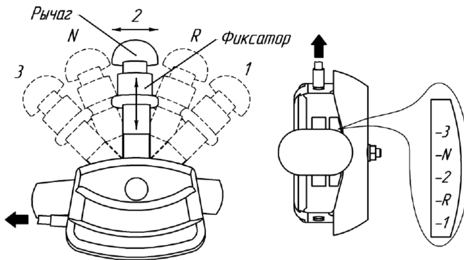
Рис.5 Рычаг переключения передач мотоблока
