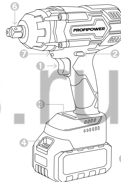
Рисунок 1.1. Устройство инструмента
